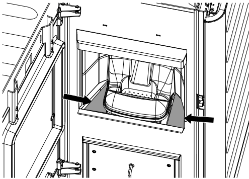
Abb. 89: Feuerraum reinigen
