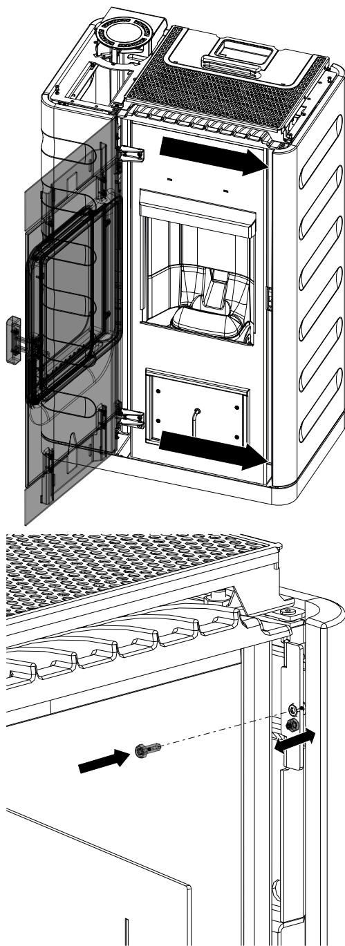
Abb. 22: Keramikverkleidung befestigen
