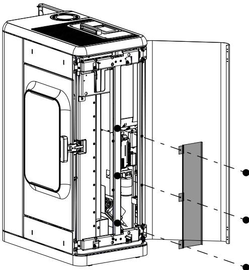
Abb. 33: Abdeckung abmontieren
