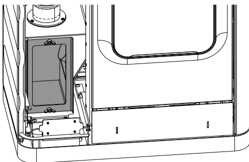
Abb. 93: Putzdeckel entfernen
