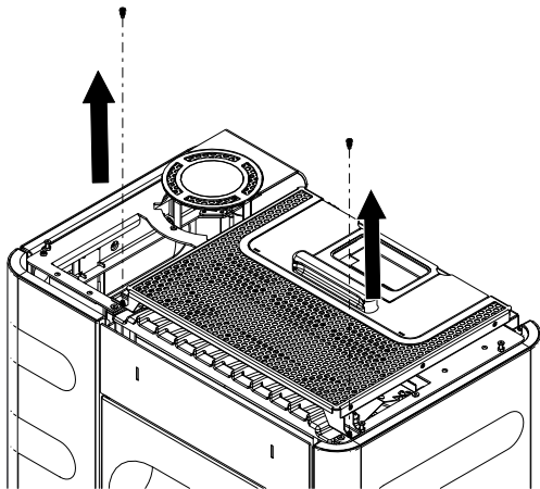
Abb. 85: Schrauben lösen
