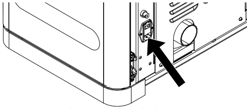
Abb. 97: Sicherungseinschub mit T2,5A-Glasrohrsicherungen
