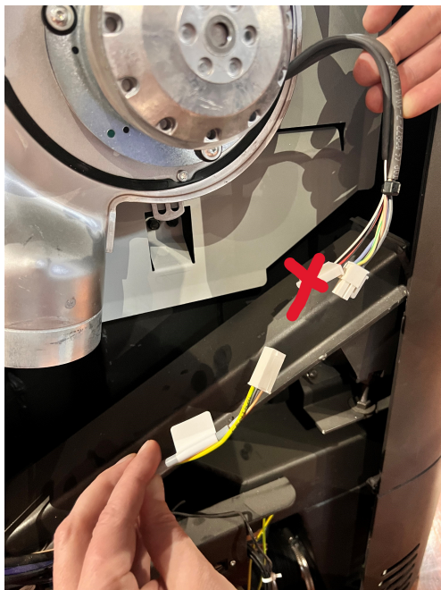
Abb. 35: Kabel verbinden
