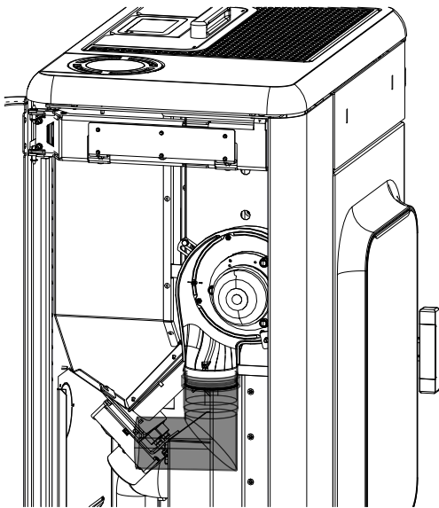
Abb. 40: Mit L-Rohrstück verbinden
