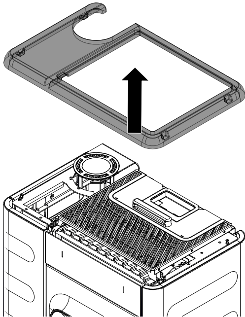
Abb. 84: Deckel abnehmen
