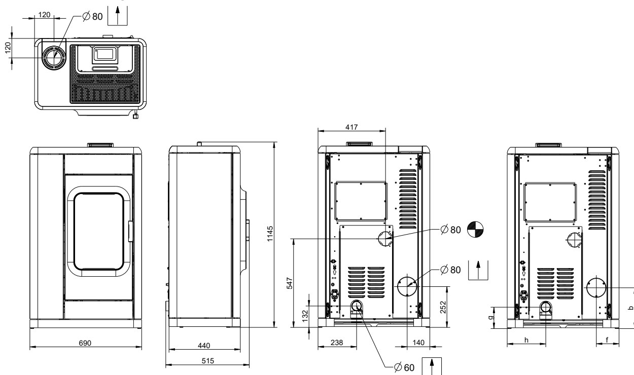
Abb. 2: Ruby Abmessungen
