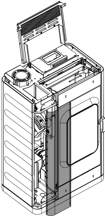
Abb. 92: Vordere Verkleidung abnehmen
