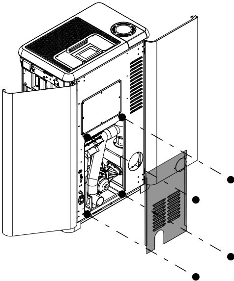
Abb. 32: Rückwand abmontieren
