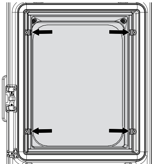
Abb. 99: Glashalter entfernen
