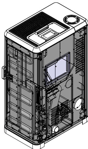
Abb. 43: Rückwand und Seitenverkleidungen montieren
