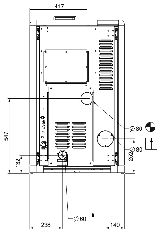
Abb. 45: Abmessungen
