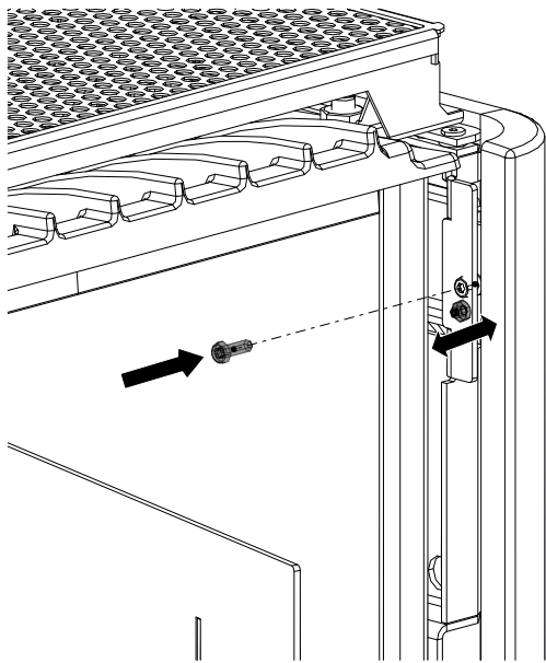
Abb. 11: Keramikverkleidung befestigen
