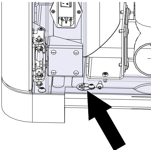
Abb. 39: Zentralerdung anschließen
