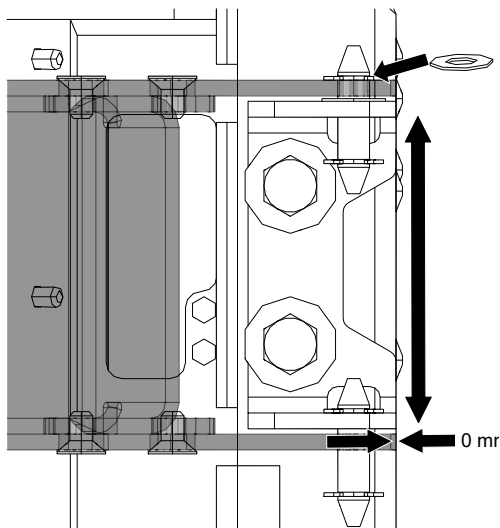
Abb. 19: Höhe der Tragarme einstellen
