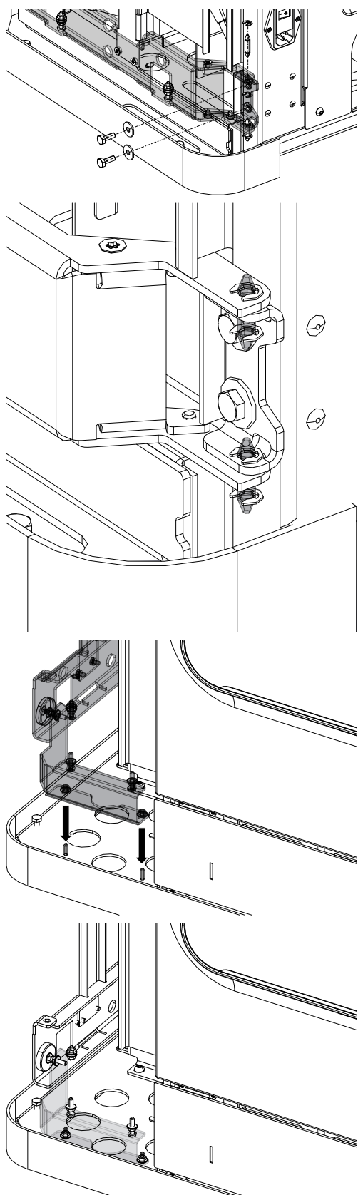
Abb. 17: Tragarme montieren
