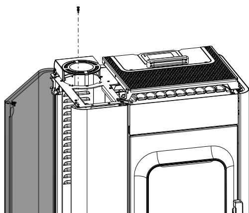
Abb. 10: Seitenverkleidung aufklappen
