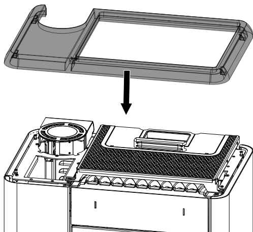
Abb. 29: Deckel anbringen
