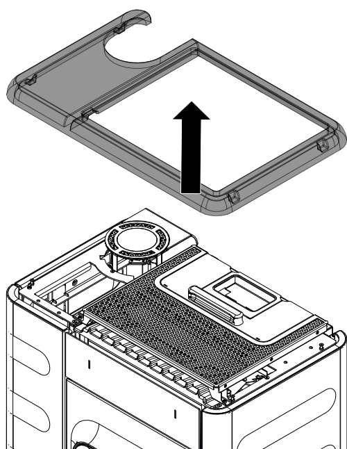
Abb. 9: Deckel abnehmen
