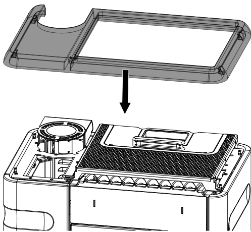
Abb. 24: Deckel anbringen
