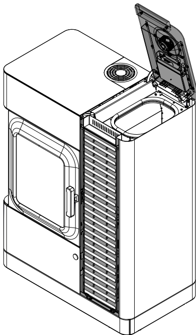
Abb. 75: Fronträger demontieren
