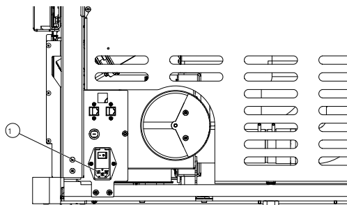
Abb. 34: Elektrischer Anschluss
