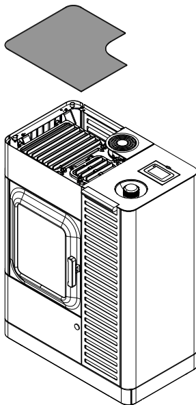
Abb. 17: Deckel abnehmen
