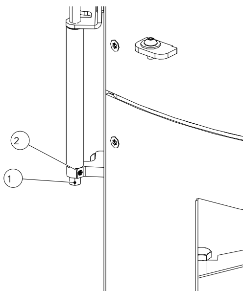
Abb. 81: Türschließkraft einstellen
