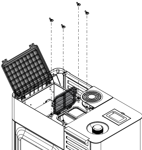
Abb. 95: Putzdeckel
