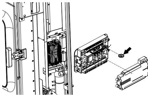
Abb. 88: Speicherbatterie tauschen
