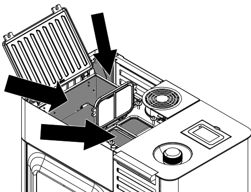
Abb. 96: Rauchgaszüge oben reinigen
