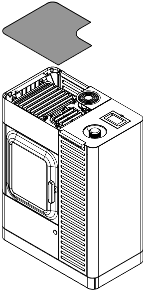
Abb. 94: Kochplatte abnehmen
