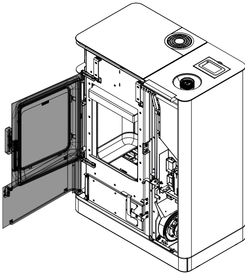
Abb. 76: Beide Türen öffnen
