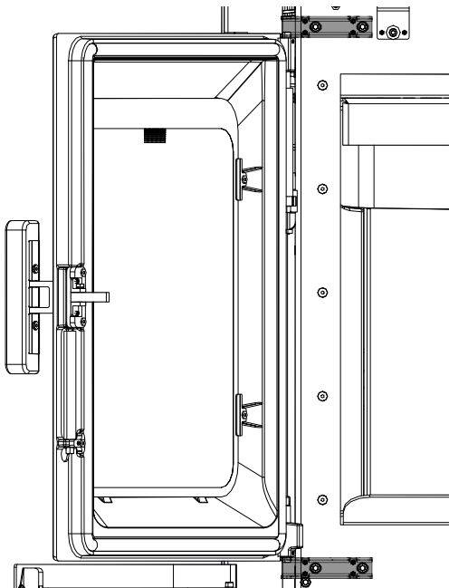
Abb. 77: Feuerraumtür einstellen
