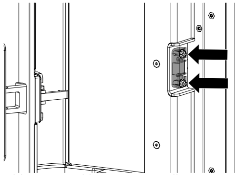
Abb. 79: Verschlussseitig einstellen
