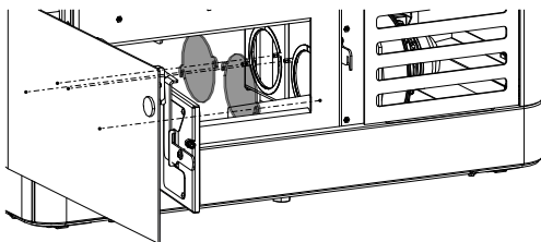
Abb. 100: Abdeckungen abmontieren
