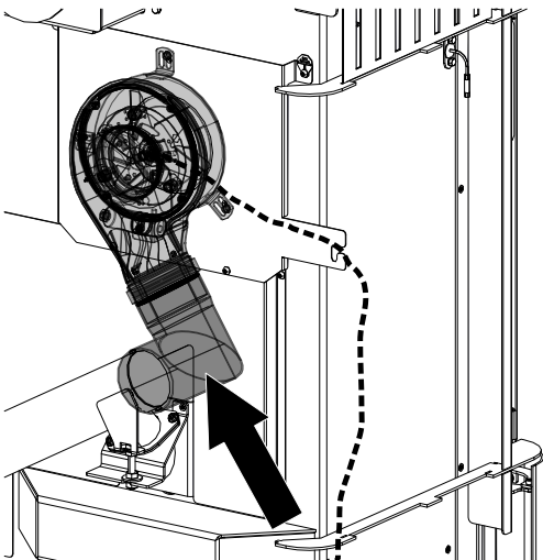
Abb. 29: Rohr raufstecken
