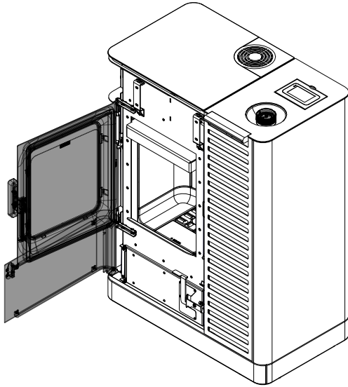
Abb. 82: Türen öffnen
