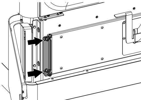
Abb. 83: Ascheladentür einstellen
