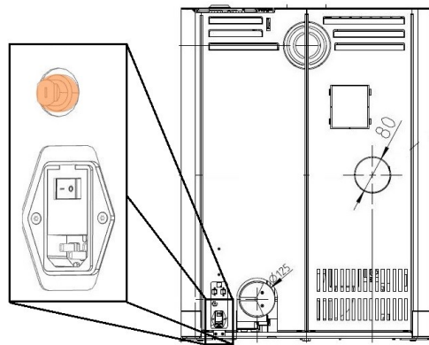
Abb. 103: Sicherheitstemperaturbegrenzer
