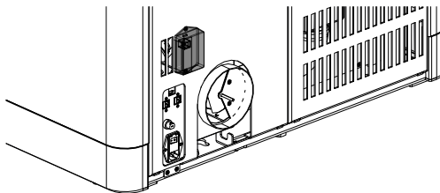
Abb. 109: WLAN-Box Abdeckung abnehmen
