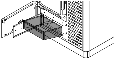
Abb. 99: Aschenlade entnehmen
