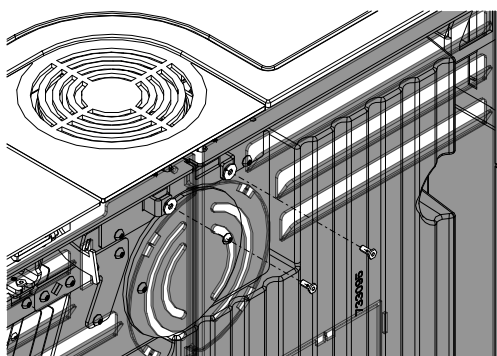
Abb. 110: Rückwand abnehmen
