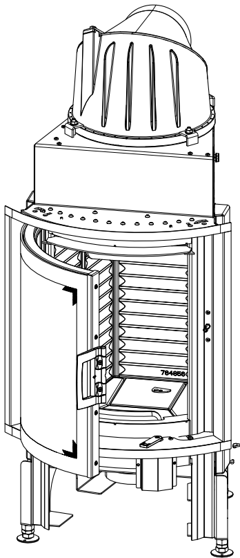
Fig. 78: Opening the door
