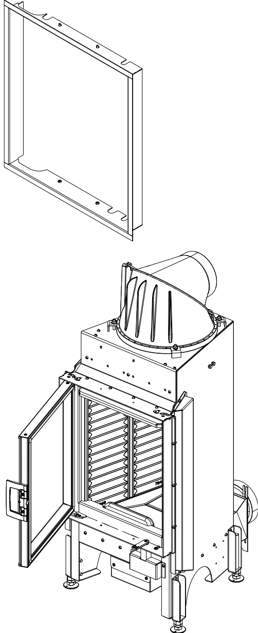
Fig. 73: Opening the door
