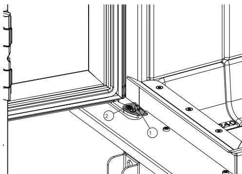
Fig. 91: Setting the door below
