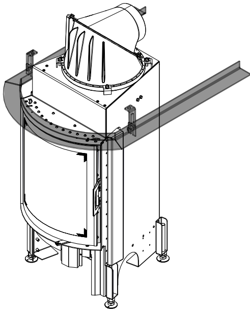
Abb. 1: Tragrahmen montieren
