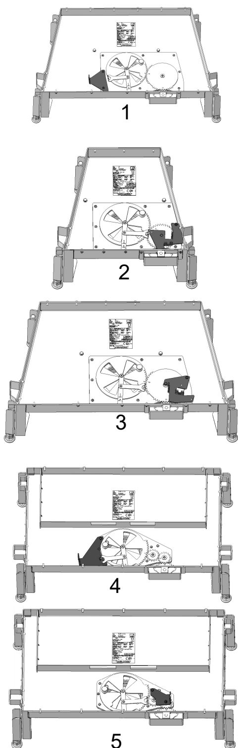
Fig. 10: Situations d'installation
