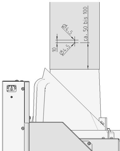
Fig. 7: Schéma de perçage pour conduit de fumée
