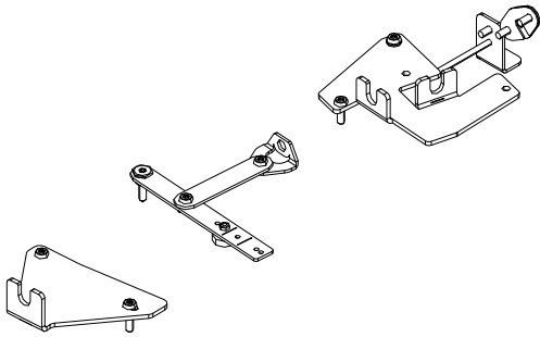
Fig. 5: Kit di montaggio 363000
