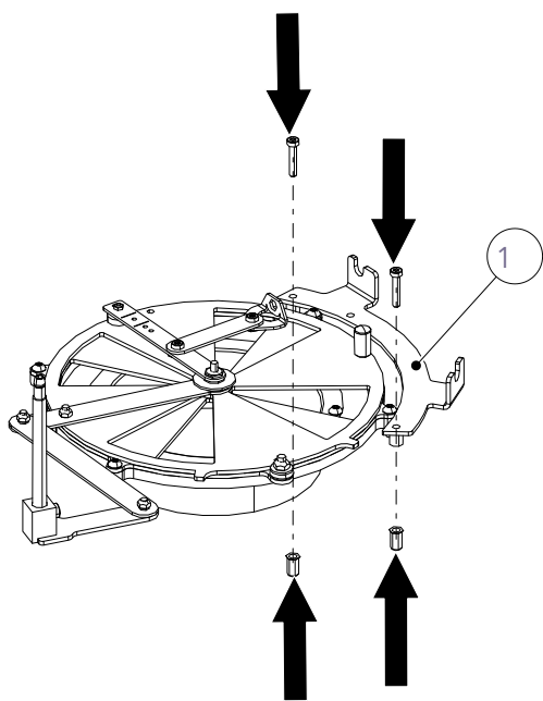
Fig. 13: Installer le kit de montage
