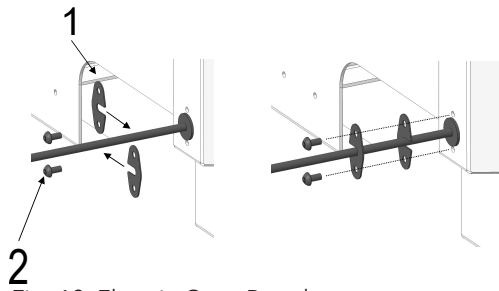
Fig. 18: Flangia Cavo Bowden
