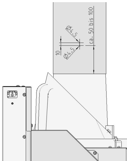
Fig. 7: Diagramma di perforazione - tubo dei fumi
