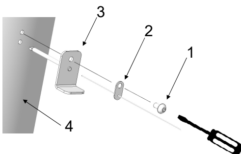
Fig. 8: Montaggio del sensore di temperatura
