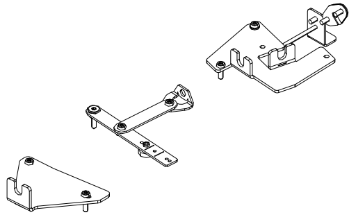
Abb. 5: Montageset 363000
