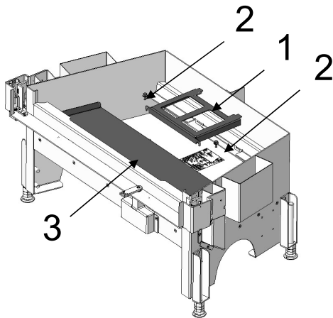
Fig. 11: Rimozione dei pezzi
