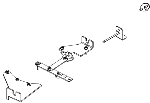
Abb. 6: Montageset 363011
