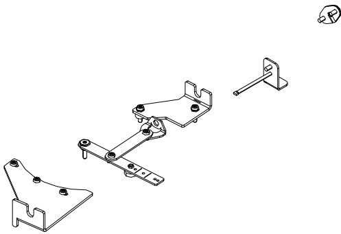
Fig. 6: Kit di montaggio 363011
