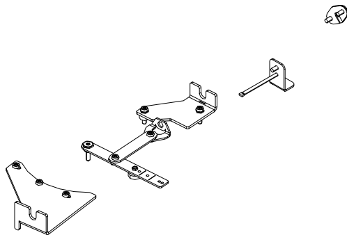
Fig. 6: Kit de montage 363011
