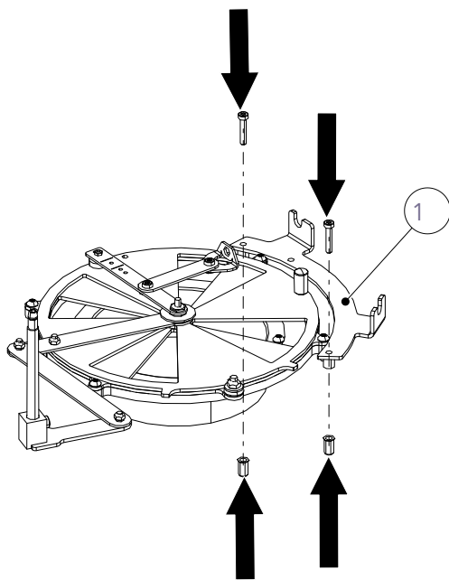
Abb. 13: Montageset montieren
