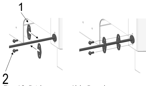
Fig. 18: Brides pour câble Bowden
