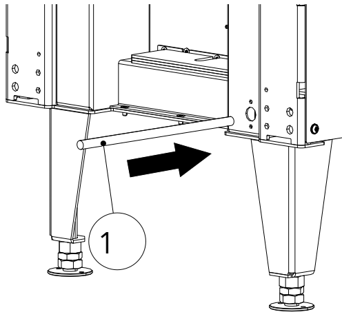
Fig. 15: Enfiler le câble Bowden
