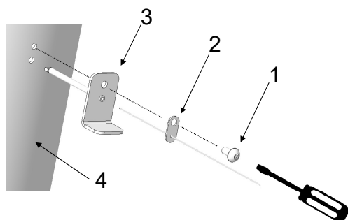
Abb. 8: Temperatur-Sensor montieren
