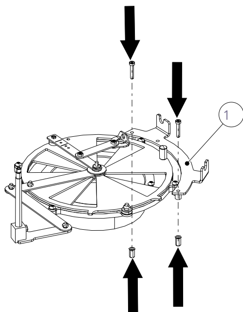
Fig. 13: Installazione del kit di montaggio
