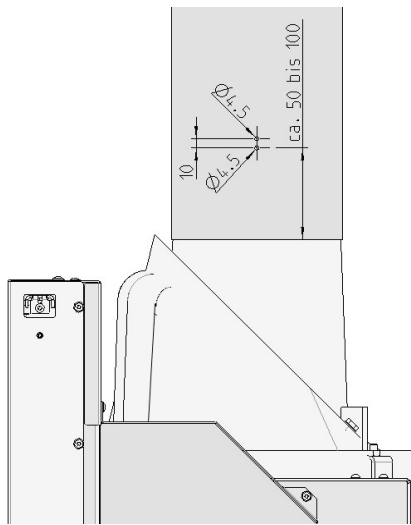
Abb. 7: Bohrschema-Rauchrohr
