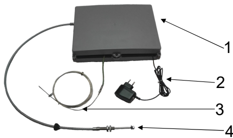
Fig. 4: Unité de contrôle
