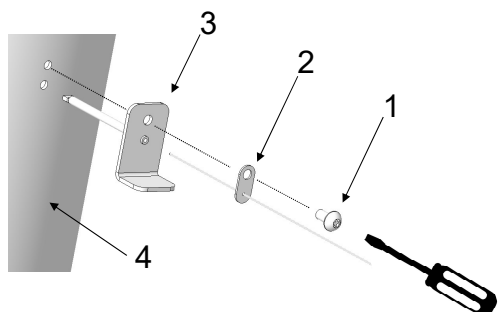
Fig. 8: Installer la sonde de température
