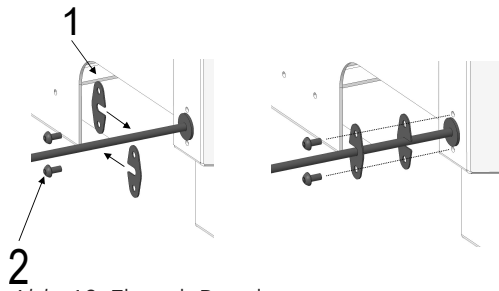
Abb. 18: Flansch Bowdenzug
