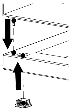
Fig. 1: Assembler le module latéral
