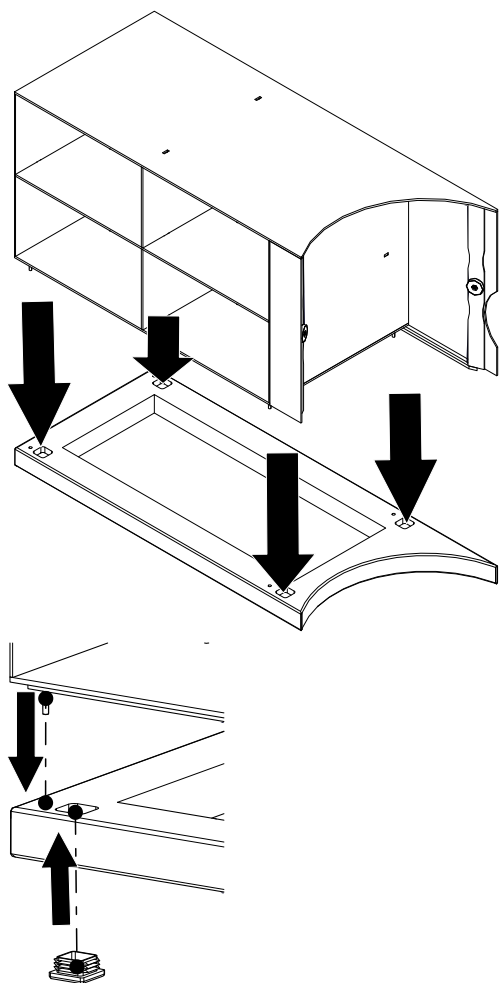
Fig. 1: Montaggio del box laterale
