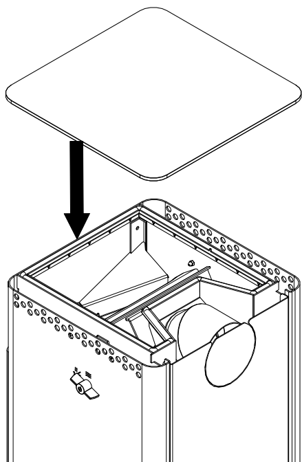
Fig. 1: Poser la plaque de cuisson
