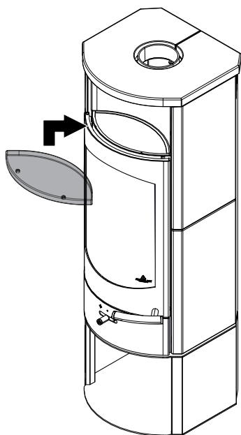
Fig. 1: Mettre en place le compartiment chauffe-plat
